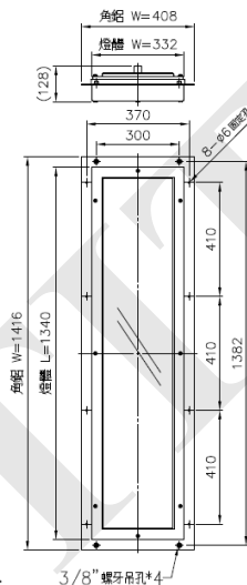
燈具尺寸-背掀
